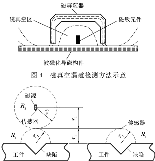
图 5 磁场扰动漏磁法与常规漏磁法对比
