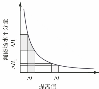
图 2 漏磁场与提离值的函数关系
