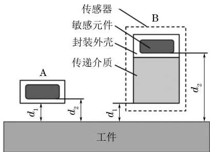
图 1 漏磁检测提离值定义示意
