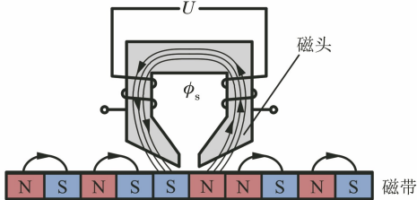
图 15 磁带磁信号拾取示意
