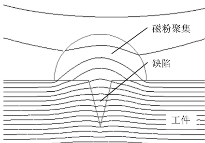
图 16 磁粉漏磁联合检测原理示意
