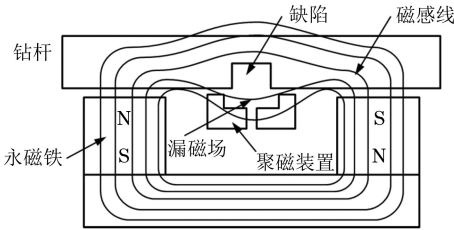
图 8 钻杆漏磁检测聚磁装置结构示意图
