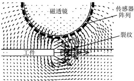
图 10 磁透镜汇聚漏磁场原理示意
